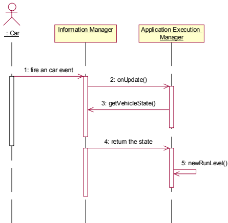
(그림 4) 차량이벤트에 따른 애플리케이션 실행 관리
