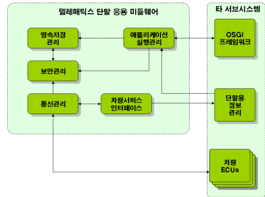
(그림 3) 미들웨어의 모듈간 연관관계
