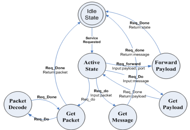
그림 4. Base Station 상태 천이도
