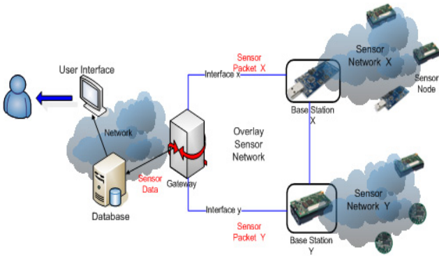
그림 2. 시스템 구조
