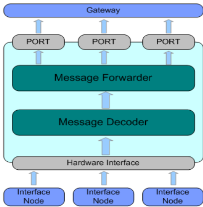
그림 3. Base Station 구조
