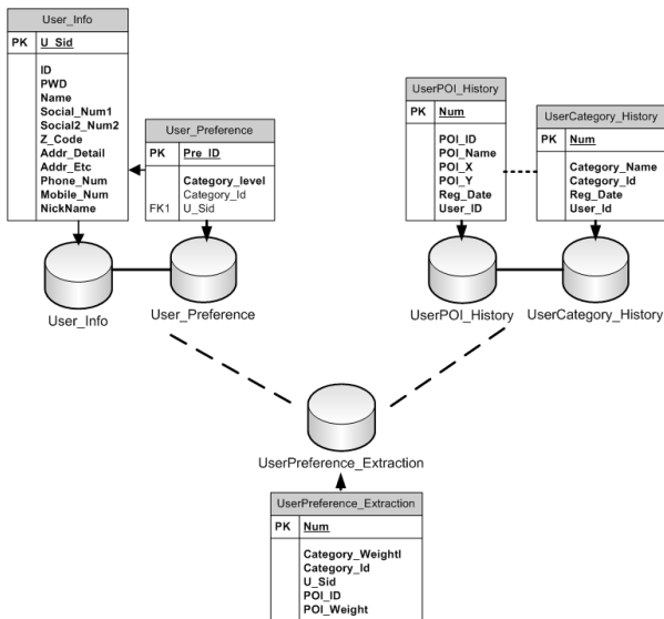
(그림 5) 사용자 선호 특성 정보 Database 스키마
