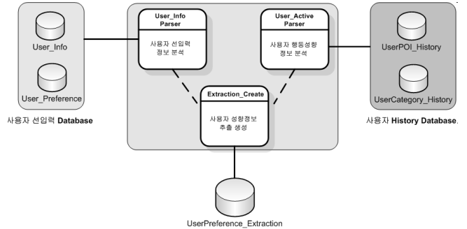
(그림 2) Monitoring Agent System 구성도
