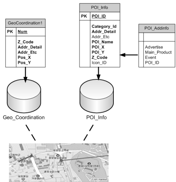
(그림 4) GIS Database 스키마
