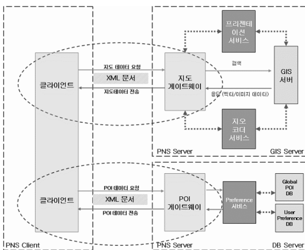
(그림 3) PNS Core 서비스 구조
