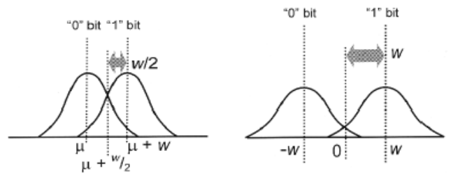
(a) 단극성 신호방식 (b) 양극성 신호방식 (그림 4) 단극성 신호방식 vs. 양극성 신호방식
