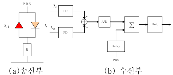
(그림 3) 송·수신부의 구조
