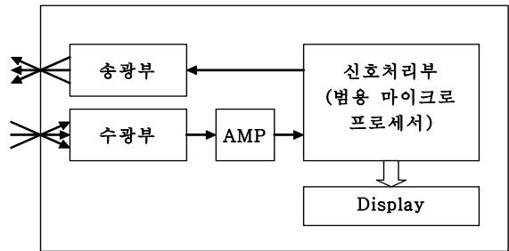
(그림 2) 제안 레이더 시스템의 블록도
