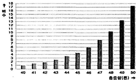
그림 1 교량 손상도(총중량 40톤을 1로 볼때)
