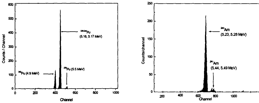
그림 3. IAEA-375 토양시료에 대한 Pu 및 Am 동위원소 알파스펙트럼
