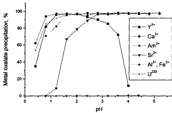
그림 2. pH변화에 따른 옥살산에 공침된 양이온들의 침전수율
