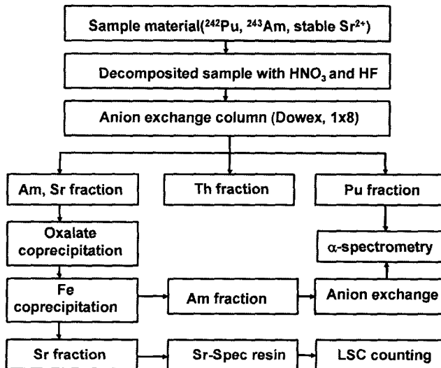
그림 1. Sr-90, Am-241 및 Pu 동위원소 측차분리 절차도
