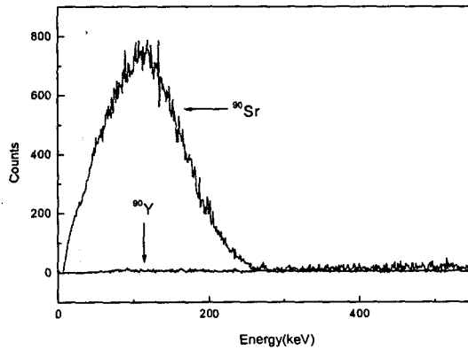
그림 4. IAEA-375 토양시료에 대한 Sr-90 및 Y-90 베타스펙트럼
