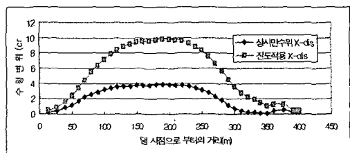
Fig. 8 3차원 진도법에 의한 변위증감도
