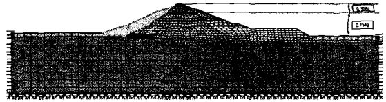
Fig. 5 수정진도법 해석모델도
