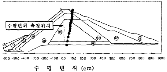
Fig. 6 수정진도법에 의한 변위 증감도
