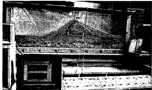
Fig. 11 진동대 시험 전경
