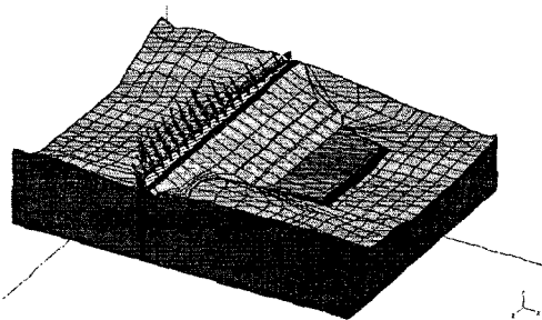
Fig. 7 3차원 등가정적 해석 모델도
