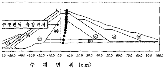
Fig. 4 진도법에 의한 변위 증감도
