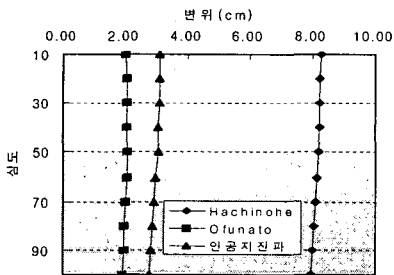
(b) 시간력응답 해석결과
