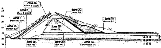
Fig. 1 해석단면
