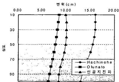
(a) 주파수응답 해석결과
