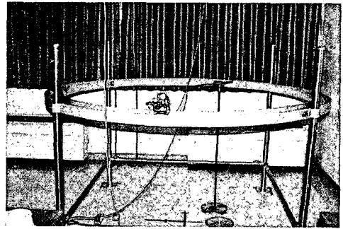
Fig. 8 원형 레일 및 구동체
