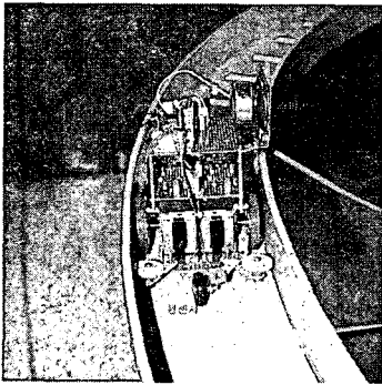
Fig.7 원형 도관으로 운행하는 바퀴달린 구동체
