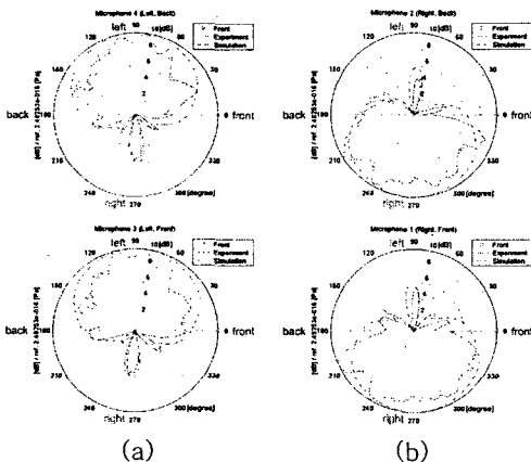
Fig. 13 2500 Hz 에서의 실험 및 시뮬레이션 결과 비교. (a) 왼쪽 (b) 오른쪽.
