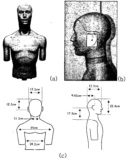
Fig. 9 Knowles 社의 KEMAR 모델
