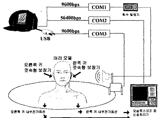
Fig.2 KEMAR 마네킹으로 실험하는 껍속형 보청기 지향성 실험 방법
