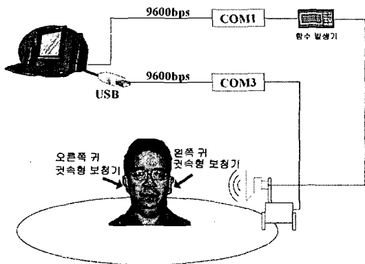
Fig.1 실제 수검자를 대상으로 실험하는 껍속형 보청기 지향성 실험 방법
