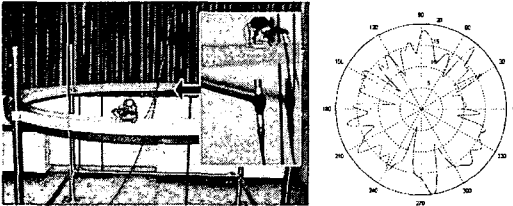
Fig. 12 원형 레일 중앙의 지향성 패턴 측정 (a) 원형 레일 중심부에 설치된 마이크론 (b) 흡음 설비를 하지 않은 측정 시스템의 중앙부 지향성 패턴
