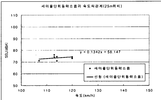
그림 7 새마을 단위 동력소음과 속도관계
