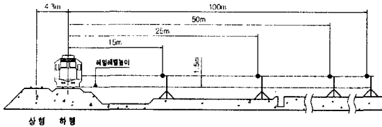
그림 4. 소음측정 현장 개념도
