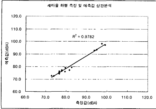
그림 13 평택-성환구간 새마을 하행 소음 상관도 분석
