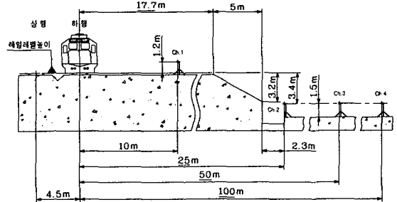
그림 11 평택-성환 구간 측정위치 단면도
