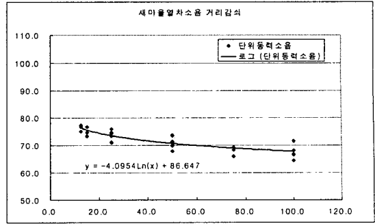
그림 9 새마을열차 단위 동력소음 SEL의 거리감쇠 특성
