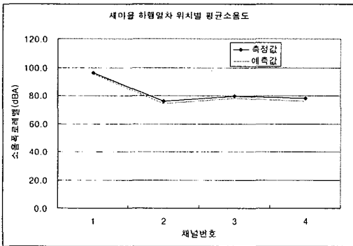
그림 15 평택-성환구간 새마을 하행선 소음도 비교
