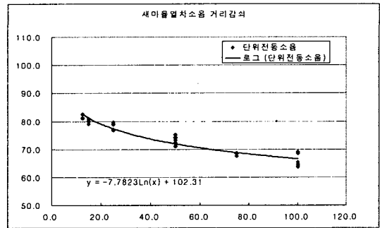
그림 10 새마을열차 단위 전동소음 SEL의 거리감쇠 특성
