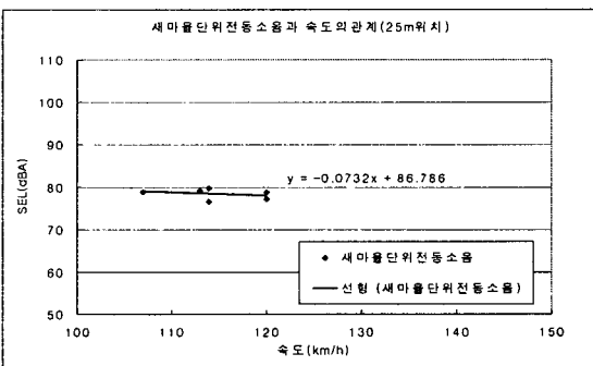
그림 8 새마을 단위 전동소음과 속도관계
