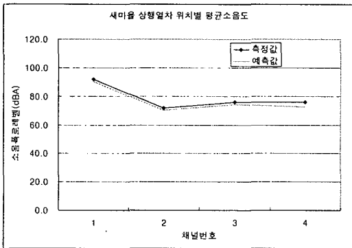
그림 14 평택-성환구간 새마을 상행선 소음도 비교
