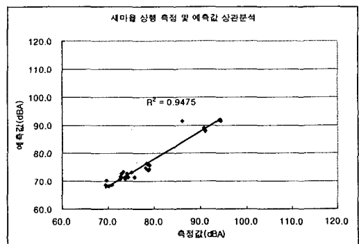
그림 12 평택-성환구간 새마을 상행열차 소음 상관도 분석
