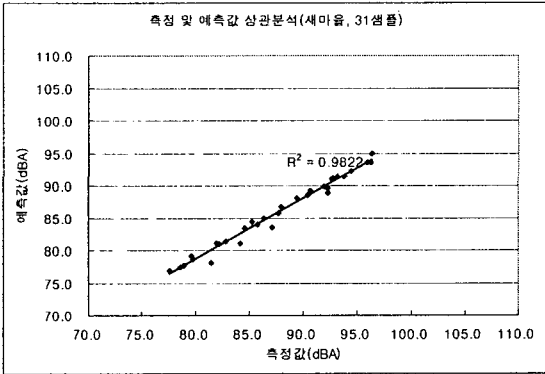
그림 6 방사소음 성분 분석값과 측정값 상관분석
