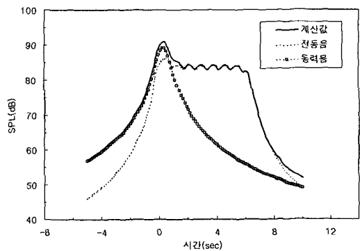
그림 3 성분 소음레벨과 합성에 의한 총 소음레벨
