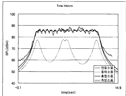
그림 5. 대표적인 성분분석 결과(대구~지천구간, 12.5m위치)
