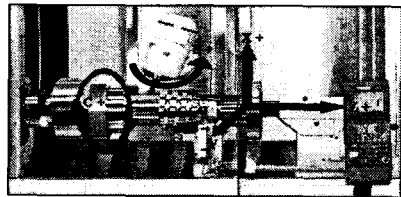
Fig. 6 Integrex-200 Mill-Turn machine
