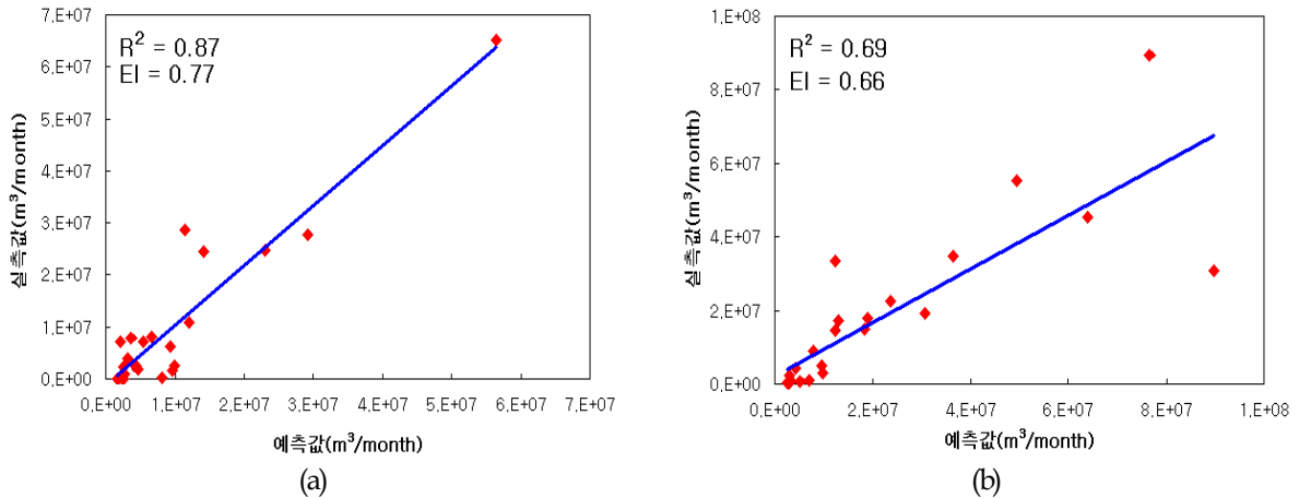
그림 4. SWAT 수문 컴포넌트의 보정 (2000~2001) (a) 과 검정 (2003~2004) (b)
