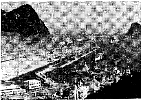
그림1) 신선대부두 축조공사
