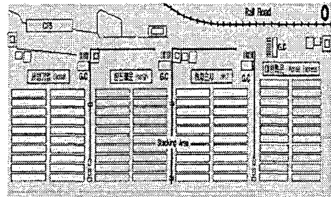
그림4) 감만 컨테이너부두 터미널 배치도
