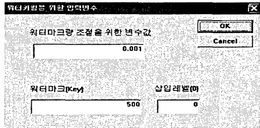
(g)워터마크 대화창
