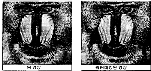
(a)원영상
