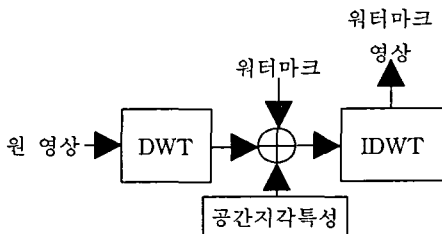
그림2. 워터마크 삽입과정
