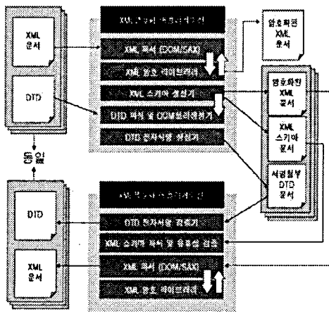
그림 3. XML 암호화 및 복호화 애플리케이션 구성도
