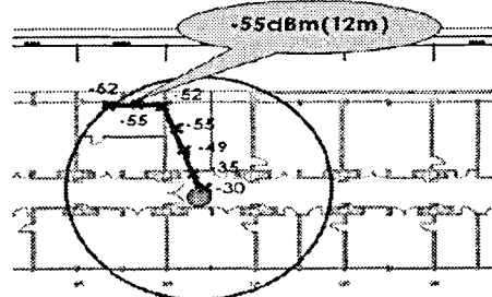
그림 7. 강의실 환경의 셀 Coverage.
