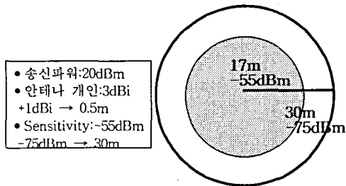
그림 5. 장애물이 없는 셀 Coverage.
