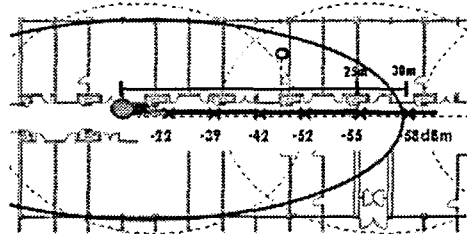
그림 6. 복도환경의 셀 Coverage.
