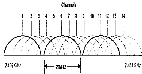
그림 4. IEEE 802.11b의 채널 구조.
