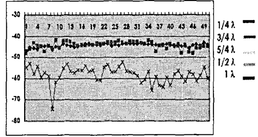
그림 14. 벽과의 이격거리 측정.
