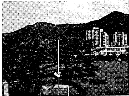
그림 1.실험에 사용된 무지향성안테나 b.급전선 LMR-400 (50Ω)
