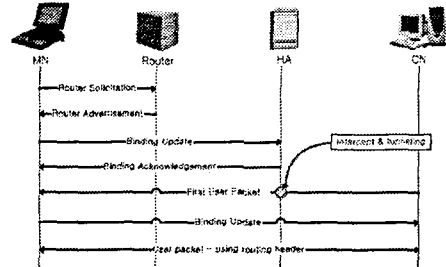
그림1. Mobile IP 메시지 흐름
