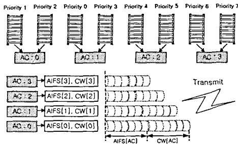
그림 3. IEEE 802.11e EDCF의 동작 과정
