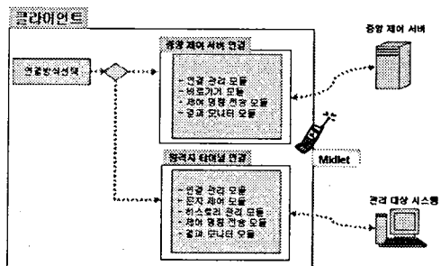
그림 2. 클라이언트 구성
