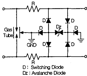
(a) 회로도
