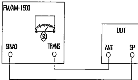
(a) SINAD 측정기 연결도 (b) SINAD measuring instrument connection
