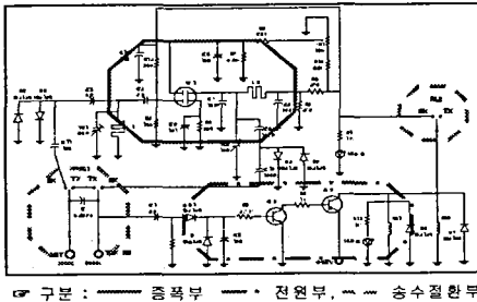
그림 1 광대역 수신증폭기 회로도 Fig 1. Broadband reception amplifier circuit
