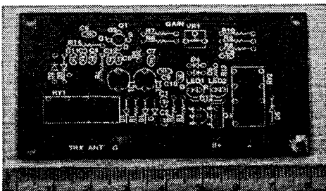
그림 2 기판상의 레이아웃 Fig 2. Layout of board
