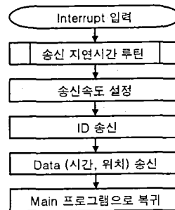
그림10 위치데이터의 송신알고리즘 Fig.10 Transmission algorithm of position data
