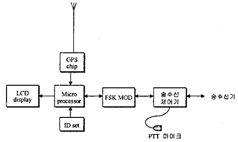
그림3 GPS-MDT 모듈의 구성도 Fig.3 Structure of GPS-MDT module
