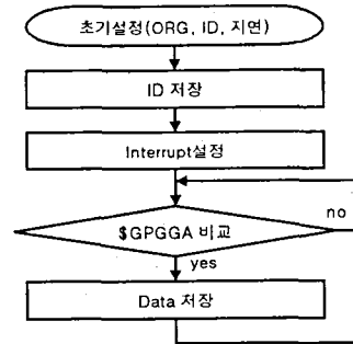
그림8 데이터의 취득알고리즘 Fig.8 Data acquisition Algorithm
