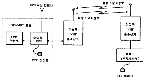
그림2 GPS-MDT의 운용 개요 Fig.2 Concept of GPS-MDT operating
