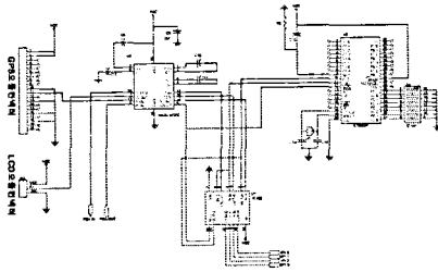
그림7 Data의 취득 및 제어부의 회로도 Fig.7 Data acquisition & control Circuit
