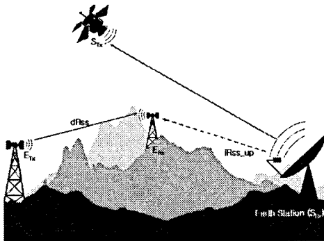
그림 2. 위성망으로부터 지상망 간섭 시나리오2
