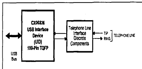
그림 6. CX06836 모뎀의 라인 인터페이스
