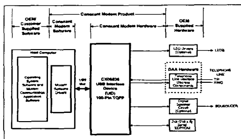
그림 7. 사용자 시스템과 CX06826 모뎀의 인터페이스
