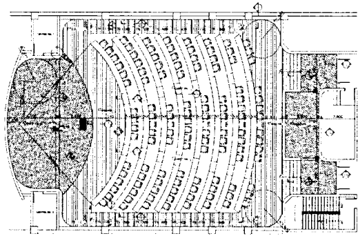
<그림 3> 강당 평면도
