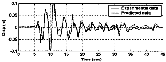
(c) 지반최대가속도가 400gal인 경우
