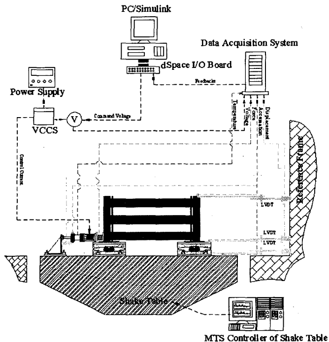
그림 1. 하이브리드 면진장치 진동대 실험의 구성도
