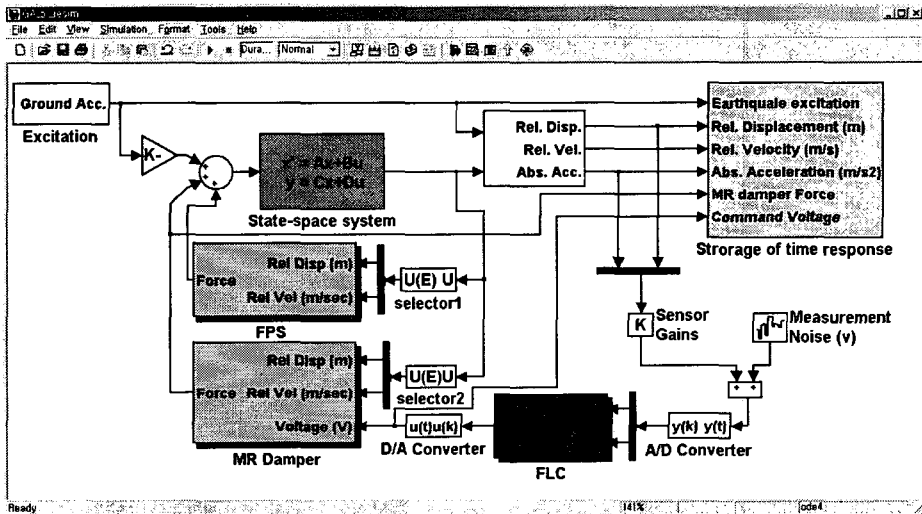
그림 7. 하이브리드 면진장치의 수치해석을 위한 SIMULINK 블록 다이어그램
