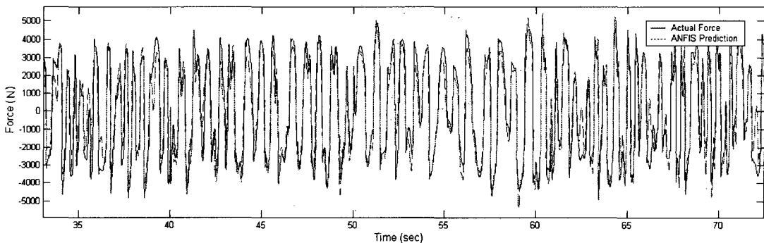
그림 2. MR 감쇠력의 성능실험 결과치와 뉴로-퍼지 모델에 의해 계산된 데이터의 비교
