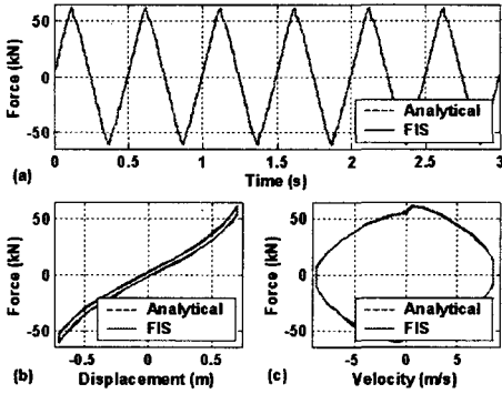
그림 4. 2 Hz 사인파 변위를 사용한 FPS 뉴로 퍼지 모델의 검증
