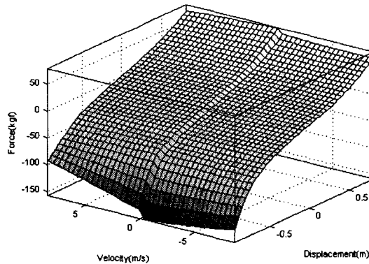
그림 3. FPS 뉴로-퍼지 모델의 rule surface
