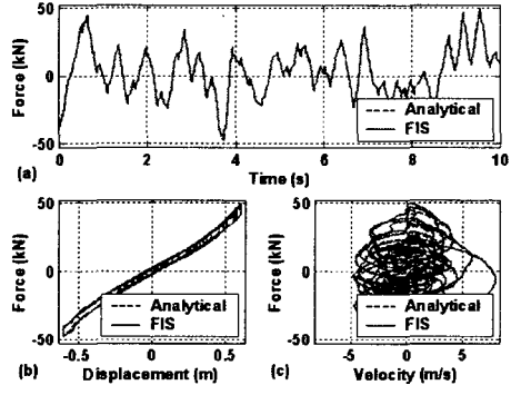
그림 5. 백색과 변위를 사용한 FPS 뉴로 퍼지 모델의 검증
