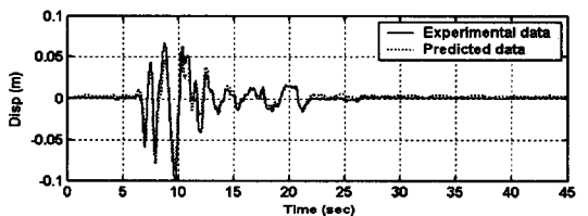
(c) 지반최대가속도가 400gal인 경우
