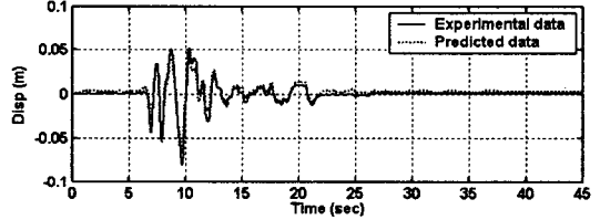
(b) 지반최대가속도가 300gal인 경우
