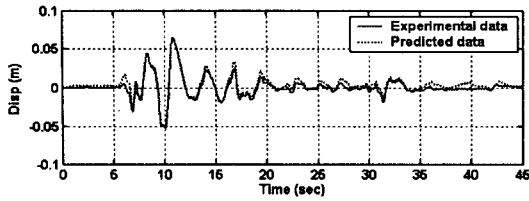
(a) 지반최대가속도가 200gal인 경우
