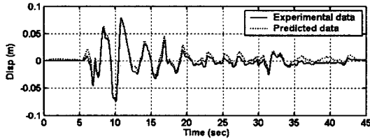
(b) 지반최대가속도가 300gal인 경우
