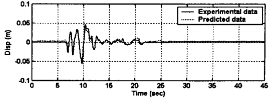
(a) 지반최대가속도가 200gal인 경우
