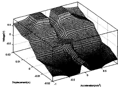
그림 6. 퍼지논리제어기의 rule surface
