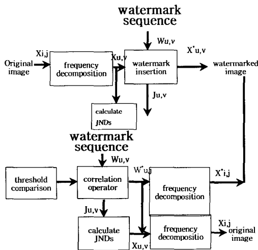
▶▶ 그림3.1 이미지 적용 워터마크의 일반적인 블록 다이어그램
