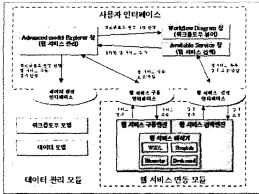
▶▶ 그림 4. One-Stop Web Services의 시스템구성도
