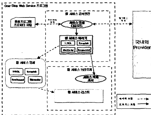
▶▶ 그림 5. Web Services 검색기능 흐름도
