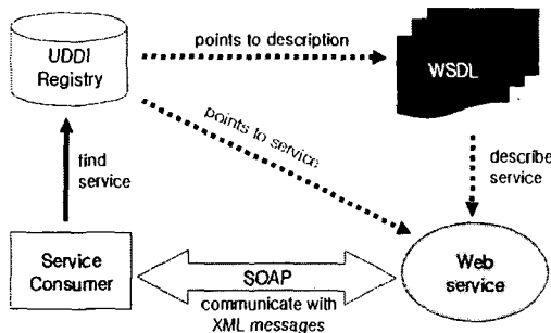
▶▶ 그림 1. Web Services의 구조
