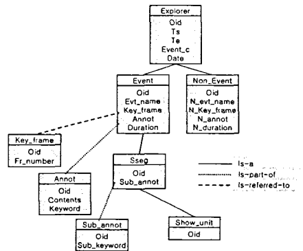
그림 2. 교양 비디오 영역의 클래스 구조
