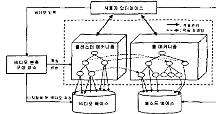
그림 3. 클러스터와 볼의 관리 구조
