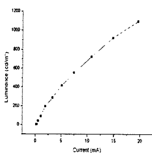
그림 2. L-I 특성 곡선
