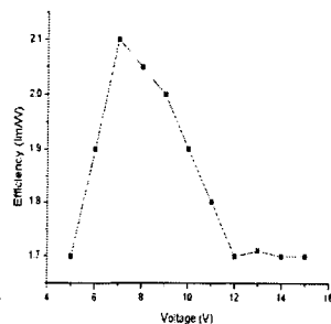
그림 3. 효율특성 곡선
