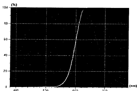
그림 4. 발광 스펙트럼
