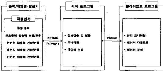
그림 5. 풍력-태양광 복합발전 모니터링 시스템 구성도
