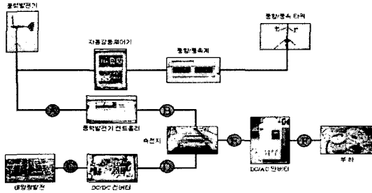
그림 1. 풍력-태양광 복합발전 시스템
