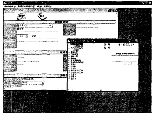
그림 8. 조명시설 관리 프로그램의 제어함 관리 기능 화면. Fig. 8. Screen of control box management for light facility management program.
