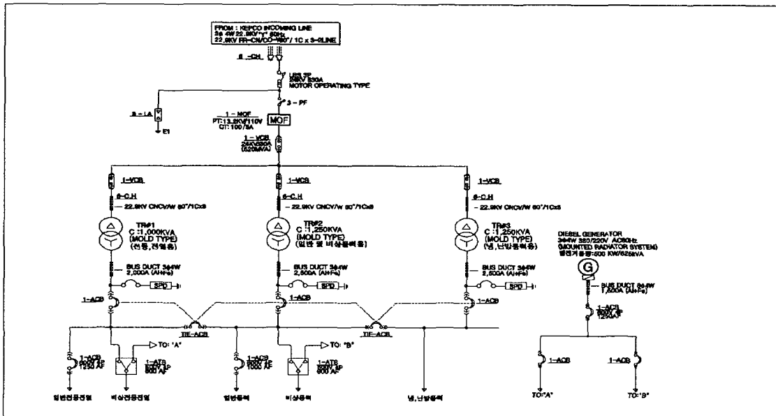
그림 2. 수변전 단선결선도
