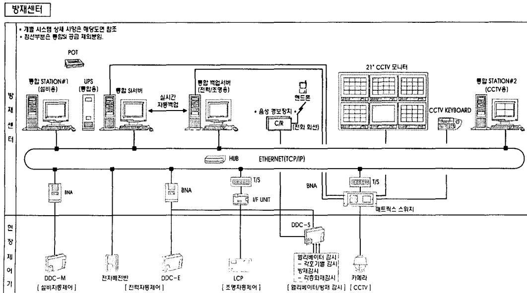
그림 6. 통합 자동제어 시스템 구성도
