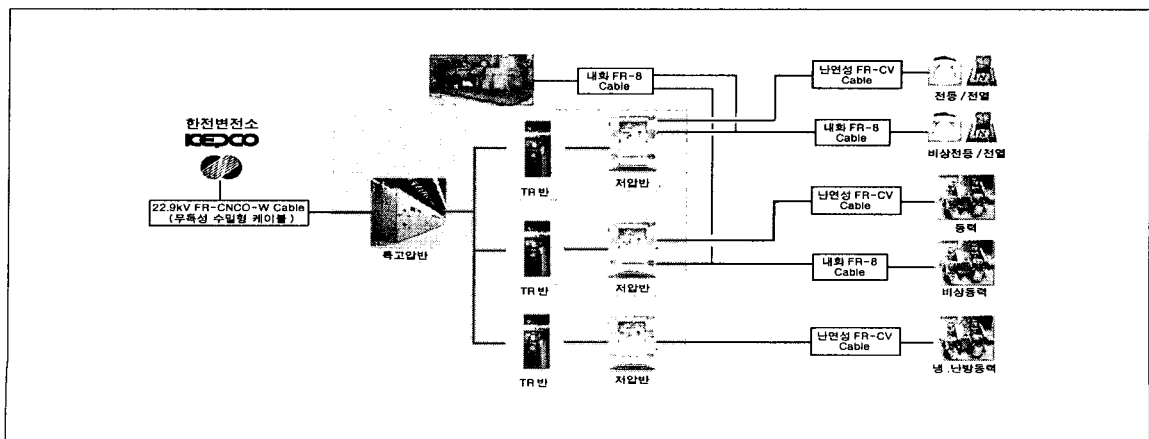
그림 4. 전력간선 구성도
