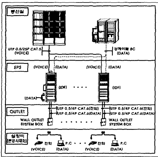
그림 7. 통합배선 구성도
