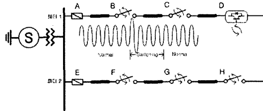
그림 4. 계통의 과도현상 발생 메커니즘 Fig.4. Voltage transient generation mechanism
