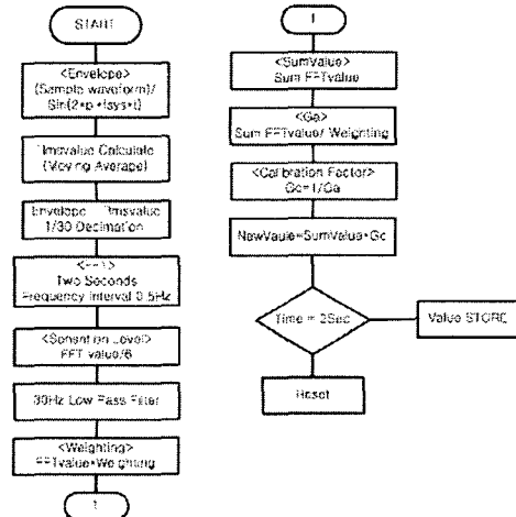
그림 5. 플리커 평가 알고리즘 Fig.5. Flicker evaluation algorithm
