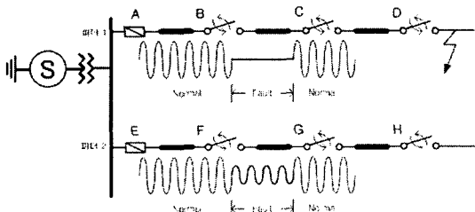
그림 3. 계통의 전압강하 발생 메커니즘 Fig.3. Voltage sag generation mechanism
