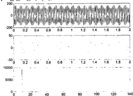
그림 6. 10Hz, 0.4pu 플리커 파형의 플리커 평가 Fig.6. Flicker evaluation of flicker waveform
