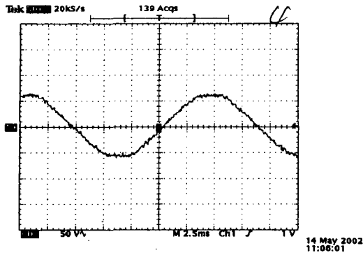
그림 7. 커먼모드 파형 Fig. 7. Common mode wave
