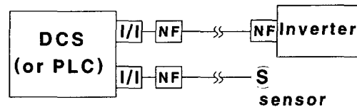
그림 13 노이즈 필터 설치 계통도 Fig. 13. Diagram by installed noise filter
