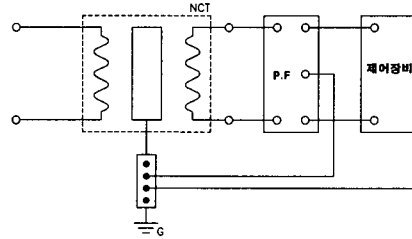
그림 5. 파워 필터와 등전위 접지를 설치한 회로도 Fig. 5. Circuit of control system installed power filter & equipotential
