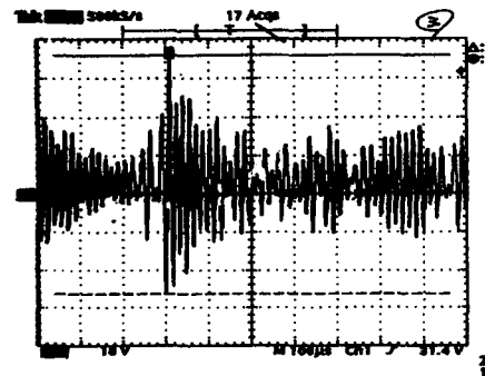
그림 12 노이즈 필터 설치전 파형 Fig. 12. Wave by un-installed noise filter
