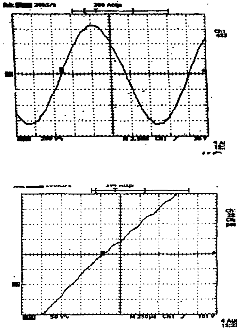
그림 11. PNR 설치후 파형 Fig. 11. Wave by installed PNR
