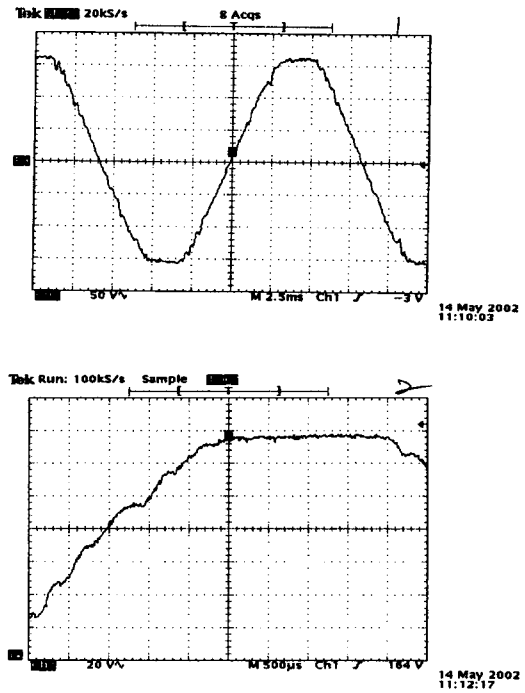
그림 6. 노말모드 파형 Fig. 6. Normal mode wave
