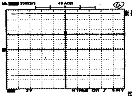
그림 14. 노이즈 필터 설치후 파형 Fig. 14. Wave by installed noise filter
