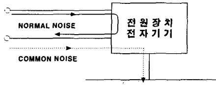
그림 1. 커먼모드 노이즈와 노말모드 노이즈 Fig. 1. Common mode noise and normal mode noise
