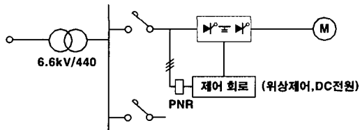
그림 8. 크레인 전원 계통도 Fig. 8. Electrical power diagram of crane
