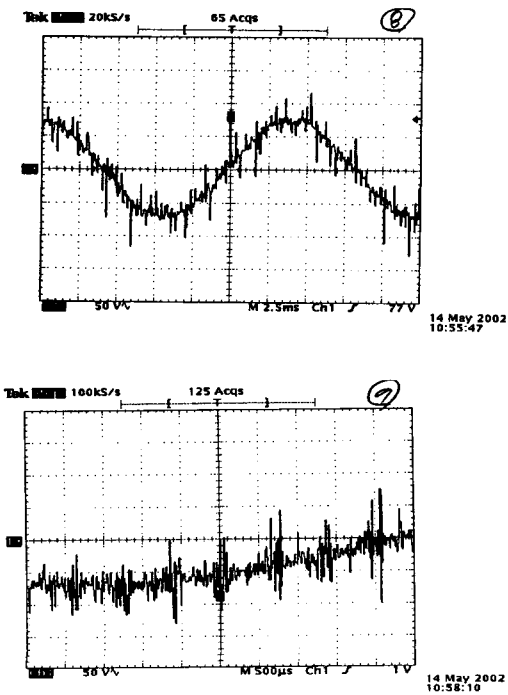
그림 6. 노말모드 파형 Fig. 6. Normal mode wave
