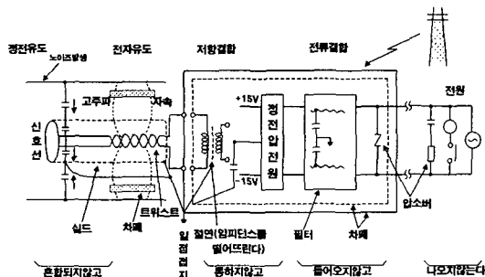
그림 2. 노이즈 장애방지 대책의 개념도 Fig. 2. Example of the noise protecting configuration
