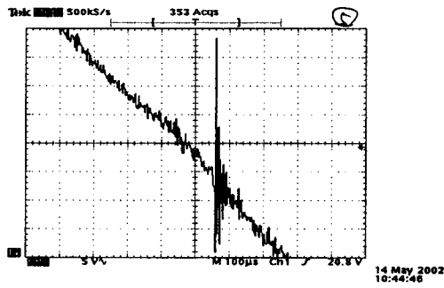
그림 3. 노말모드 노이즈 파형 Fig. 3. Normal mode noise wave
