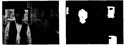
그림 4. CCD 컬러 영상에서 Cb,Cr 값을 이용한 얼굴 후보 영역 추출의 문제점. (a) 얼굴 영역의 Cb, Cr 값과 유사한 색원이 존재하는 영상. (b) (a)의 영상에 그림 3의 얼굴 후보 영역 추출 알고리즘을 수행한 결과.
