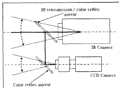
그림 5. 컬러 영상 및 적외선 영상 동시 획득 장치.
