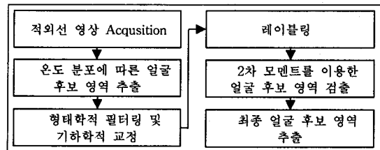
그림 1. 적외선 영상에서의 얼굴 후보 영역 추출 알고리즘.
