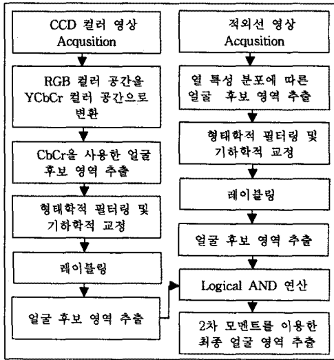
그림 6. 적외선 영상과 CCD 컬러 영상의 논리합을 이용한 얼굴 영역 추출 알고리즘.
