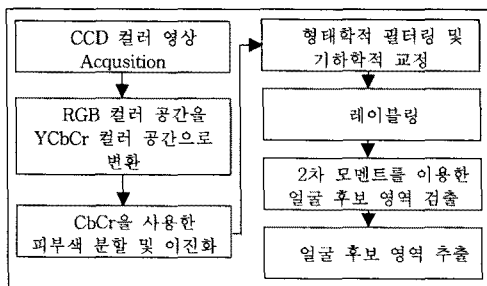
그림 3. CCD 컬러 영상에서의 얼굴 후보 영역 추출 알고리즘.
