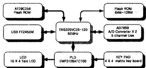
그림 1 시스템 블록도
