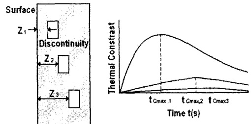
그림 1 결함깊이에 대한 열적대비[2]
