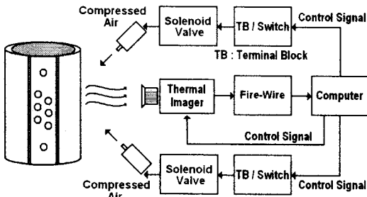
그림 4 냉각법 설비구성도
