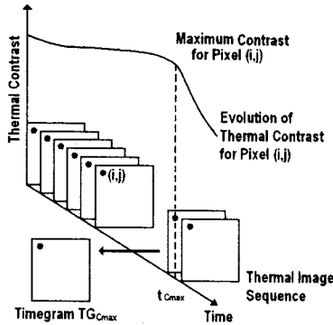
그림 2 연속 열화상에서의 시화상
