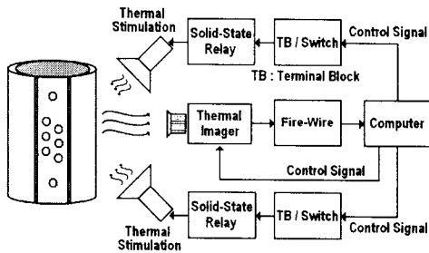
그림 3 열인가법 설비구성도
