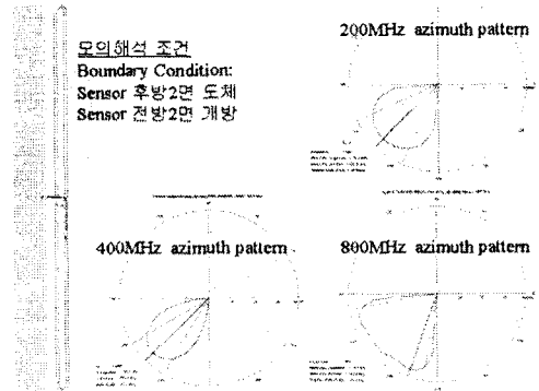
그림 3. 설계한 센서의 유증 azimuth 방사패턴
