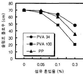
그림 3. 섬유 혼입률에 따른 슬럼프 플로우
