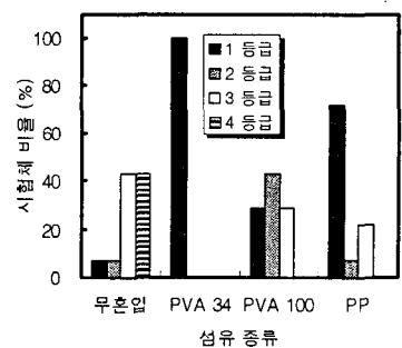
그림 5. 각섬유를 0.1% 혼입한 시험체의 폭열성상
