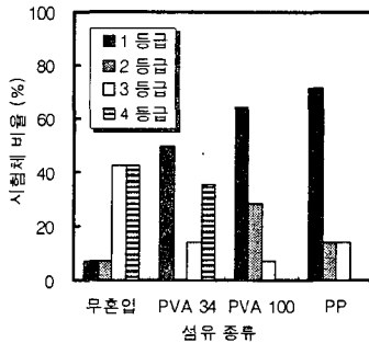
그림 4. 각섬유를 0.05% 혼입한 시험체의 폭열성상
