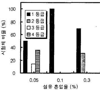
그림 6. PVA 34 \mu m 섬유를 혼입한 시험체의 폭열성상
