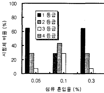
그림 7. PVA 100 \mu m 섬유를 혼입한 시험체의 폭열성상
