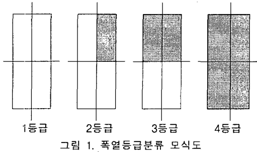
그림 1. 폭열등급분류 모식도
