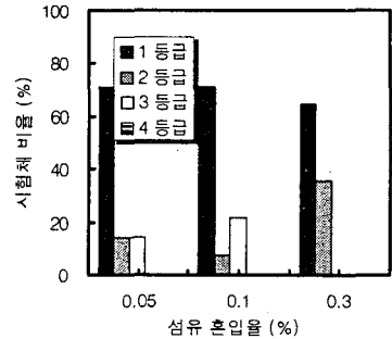
그림 8. PP 40 \mu m 섬유를 혼입한 시험체의 폭열성상
