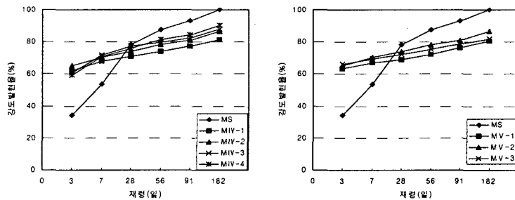
d. 온도상승구배와 압축강도의 관계
