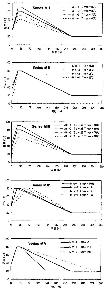
그림 1 온도이력조건
