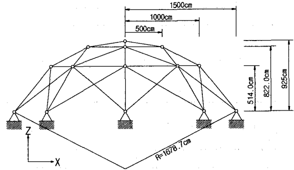
〈그림 14〉 공간 트러스 돔의 입면도
