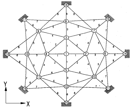
〈그림 13〉 공간 트러스 돔의 평면도
