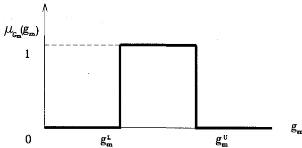
<그림 3> 보통함수의 소속함수
