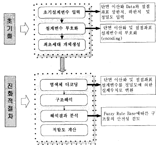
<그림 5> FGAs 알고리즘
