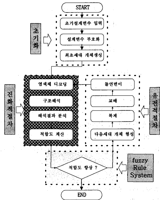
<그림 4> FS-GAs 적용 흐름도
