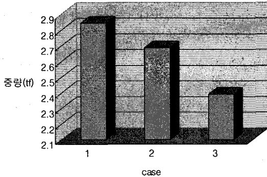
〈그림 15〉 공간 트러스돔의 목적함수비교 case 1 : 형상 고정 (비퍼지) case 2 : 형상 고려 (비퍼지) case 3 : 형상고려 (퍼지 허용오차10%범위)
