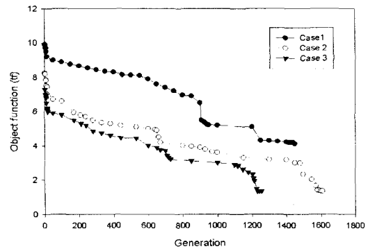
〈그림 12〉 외렌 평면 트러스의 목적함수 변화
