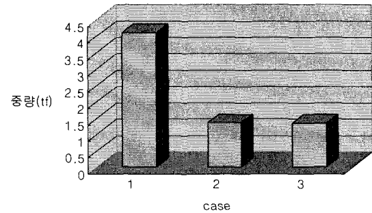
〈그림 11〉 19부재 외렌 평면 트러스의 퍼지상태에 따른 형상최적설계의 목적함수비교
