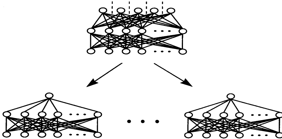
<그림 2> 신경회로망의 분리
