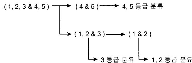
<그림 3> 이진 분류 모형의 등급 결정과정
