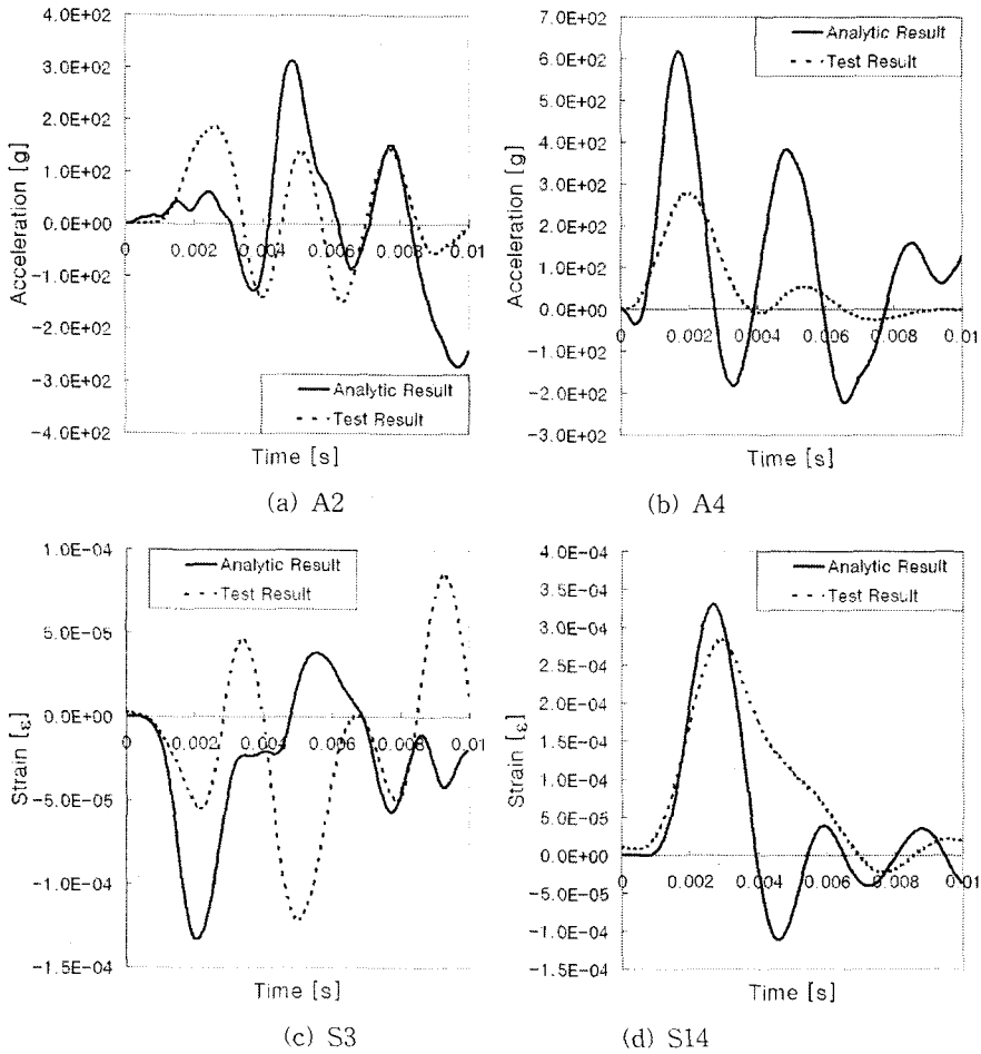
그림 12. 1/3시험모델 전복사고조건에서 해석결과와 시험결과와의 비교.
