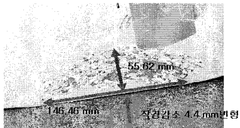
그림 9. 1/3시험모델의 전복시험 이후 뚜껑 충격 부근의 영구변형.
