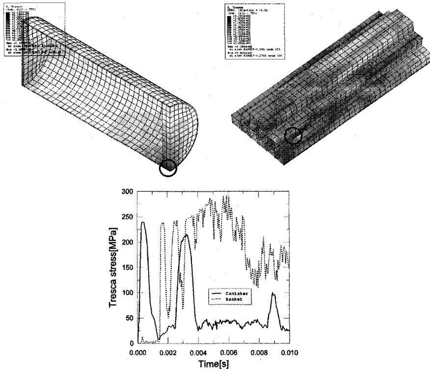
그림 6. 1/3시험모델 전복해석에서 최대 Tresca 응력선도
