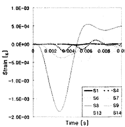
(a) 취득한 변형률
