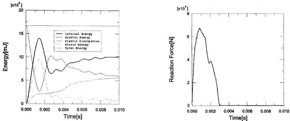
그림 5. 1/3시험모델 전복해석에서 에너지선도와 반력선도.
