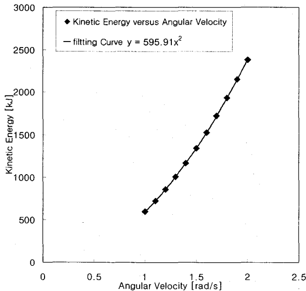
그림 3. 저장용기 본체 모델에 대한 각속도에 따른 최대 운동에너지.
