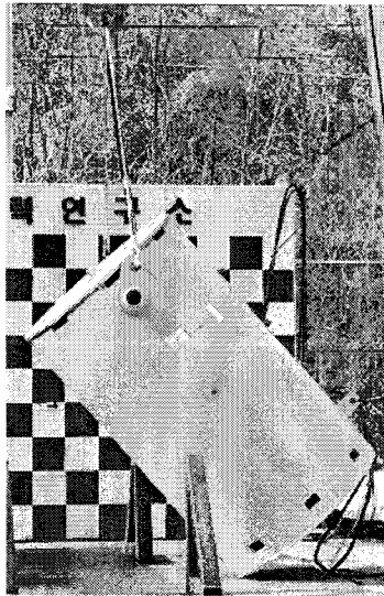
그림 8. 시험모델의 전복시험.
