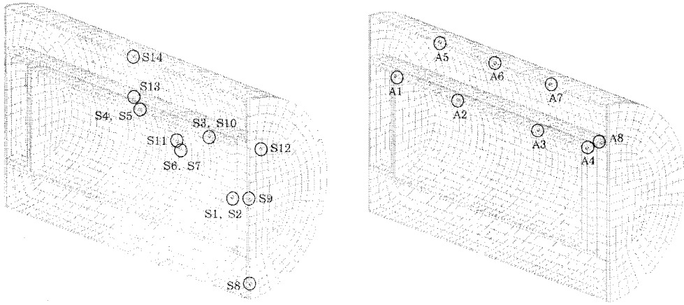
그림 7. 1/3시험모델의 전복시험에서의 센서위치
