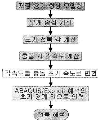
그림 1. 전복해석 순서도.
