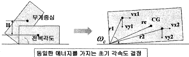
그림 2. 전복해석 초기속도를 결정하는 개념도.
