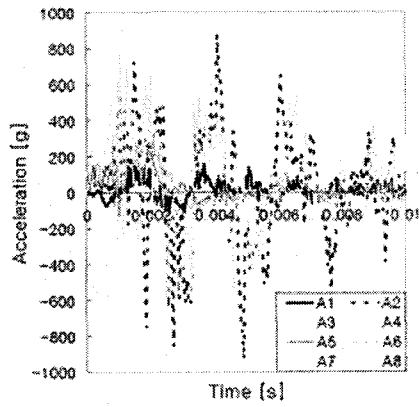
(d) 300 Hz Lowpass Filtering 가속도
