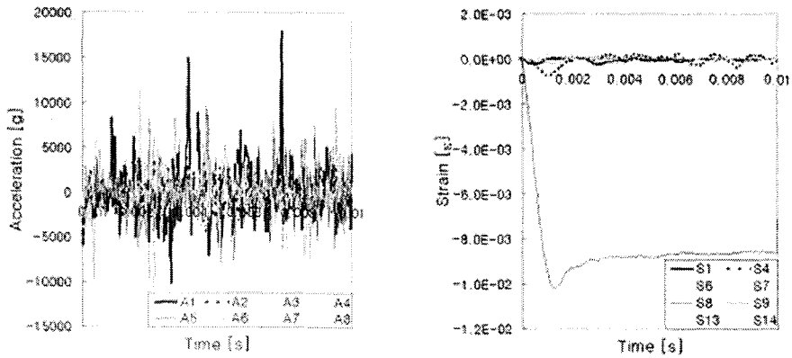
그림 11. 1/3시험모델 전복시험의 센서위치에서의 해석결과.
