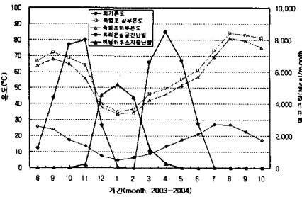
Fig. 8 월별 축열조온도 및 난방공급열량 비교
