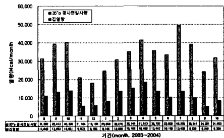
Fig. 2 월별 총 일사량 및 전체 집열량 분포 (전체 집열면적: 331.28m 2 )
