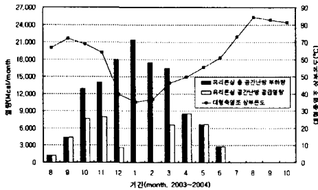
Fig. 10 월별 유리온실 공간난방부하 대비 공간 난방 공급열량 비교
