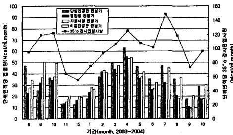
Fig. 4 월별 집열기 유형별 단위면적당 집열량 및 일사량 분포
