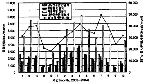
Fig. 3 집열기 유형별 집열량 및 일사량 분포 (단일진공관형:56m 2 , 평판형:69.6m 2 , 지붕형:55.68m 2 , 이중진공관형:150m 2 )
