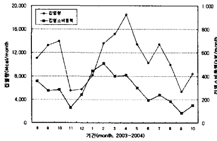
Fig. 7 월별 집열량 및 집열소비동력 비교
