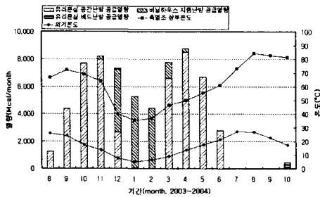
Fig. 9 월별 수요처에 따른 난방공급열량 비교
