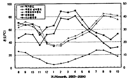
Fig. 6 월별 외기온도, 축열조상.하온도, 집열효율, 시스템효율 비교
