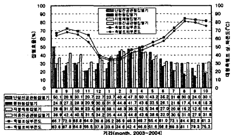
Fig. 5 월별 집열기 유형별 집열효율 비교
