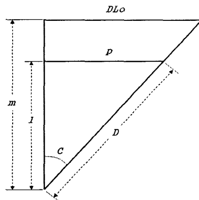
Fig. 7 Mercator sailing
