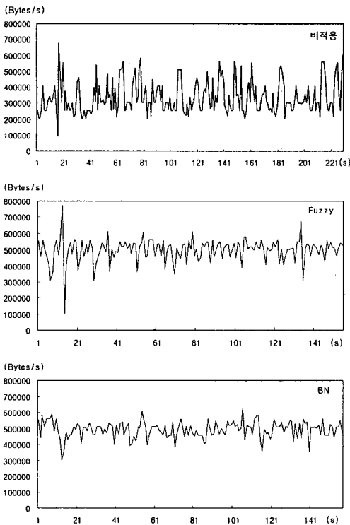
그림 6. 각 미들웨어를 적용한 응용 프로그램의 데이터 전송량
