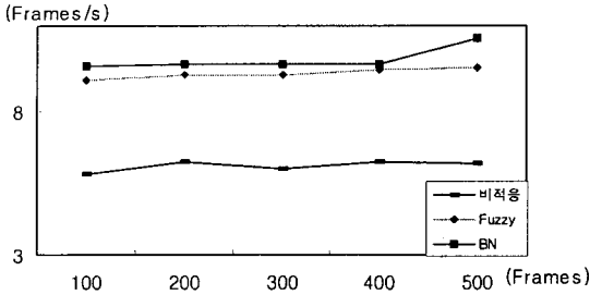
그림 5. 100~500 Frames 당 평균 프레임율
