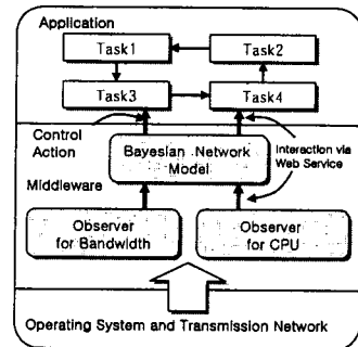
그림 1. 미들웨어 컨트롤 프레임워크 컴포넌트
