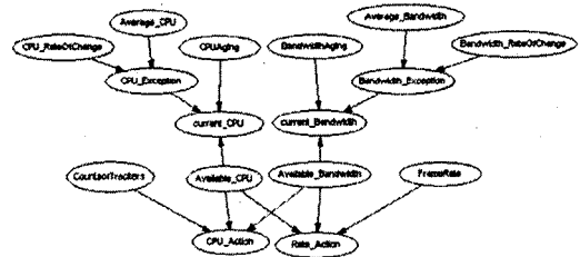
그림 4. 적응 행동을 예측하기 위한 베이저안 네트워크
