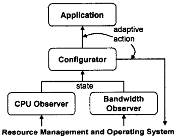
그림 3. 미들웨어 컨트롤 프레임워크 컴포넌트
