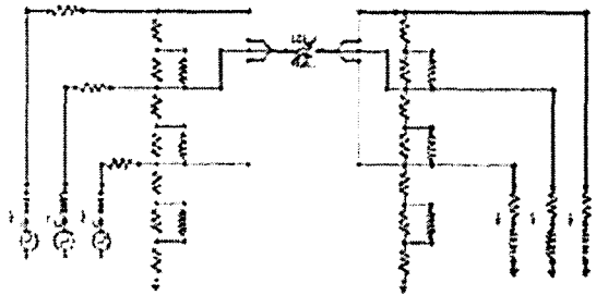
<그림-1 : 등가모델>
