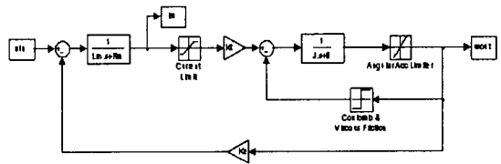
그림 2. 직류모터의 동특성 모델
