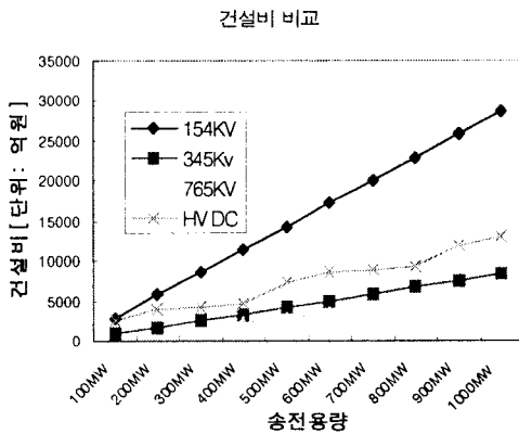
그림 2. 송전용량에 따른 송전선 건설비 비교(100Kkm)
