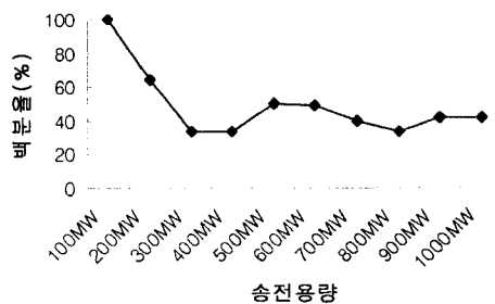
그림 3. 송전용량의 증가에 따른 건설비차 비율(%)
