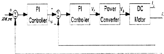
그림 4. 제어기 구성도
