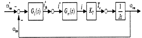
그림 2. 속도제어기
