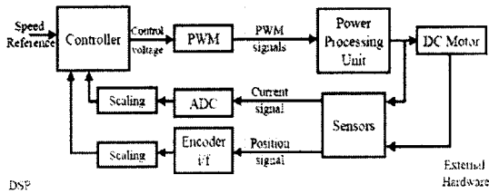
그림 3. 전체 시스템 구성도
