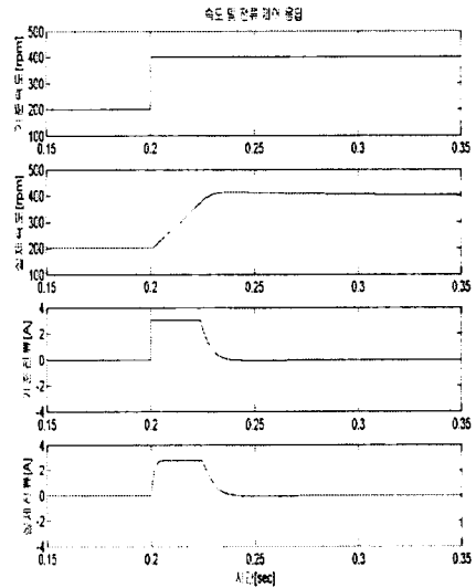
그림 6. 가속시 스텝응답(200→400RPM)
