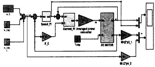
그림 5. 시뮬레이션 제어블록
