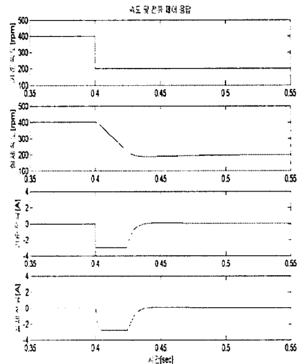
그림 7. 감속시 스텝응답(400→200RPM)
